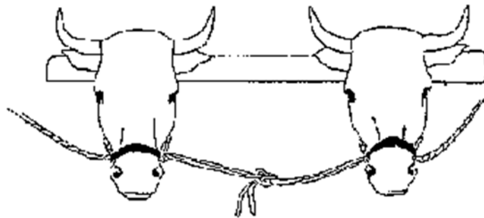
Fig. 6: OUI! La corde de joint des têtes et la corde de direction sont correctement ajustées.
