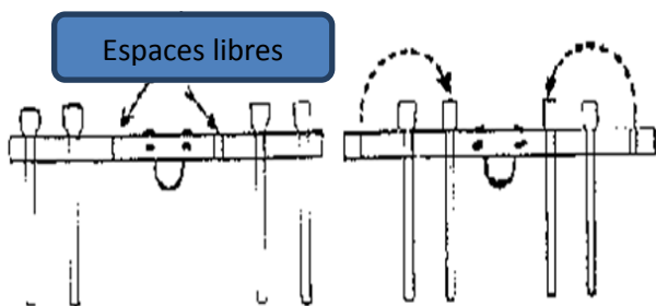
Fig. 10: Utiliser le joug long pour le billonnage, désherbage et le moulage.
